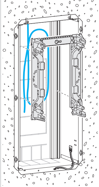
En bac d'encastrement
