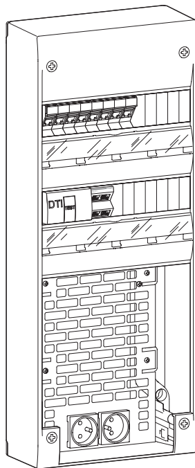
TN131 Répartiteur téléphonique 1 x 4 sorties
