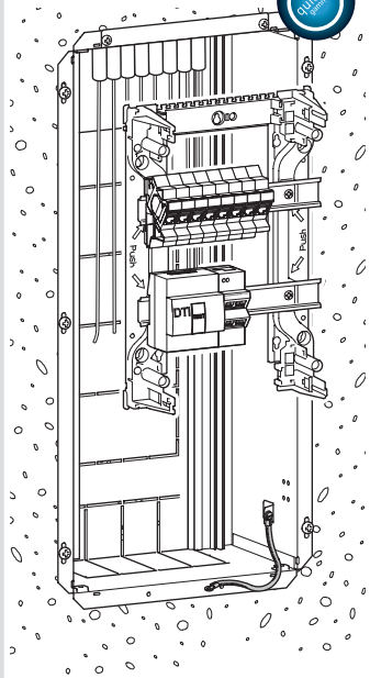
Pose en bac d'encastrement
