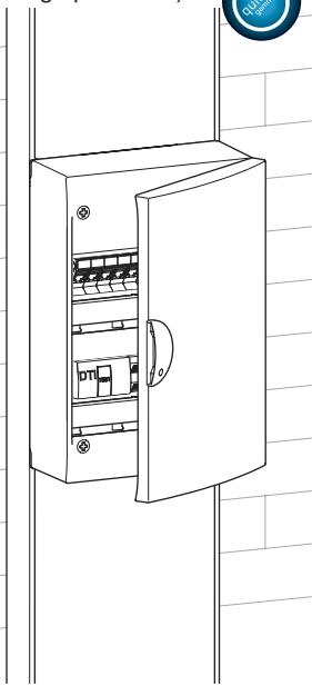
Pose sur goulotte (montage préconisé)
