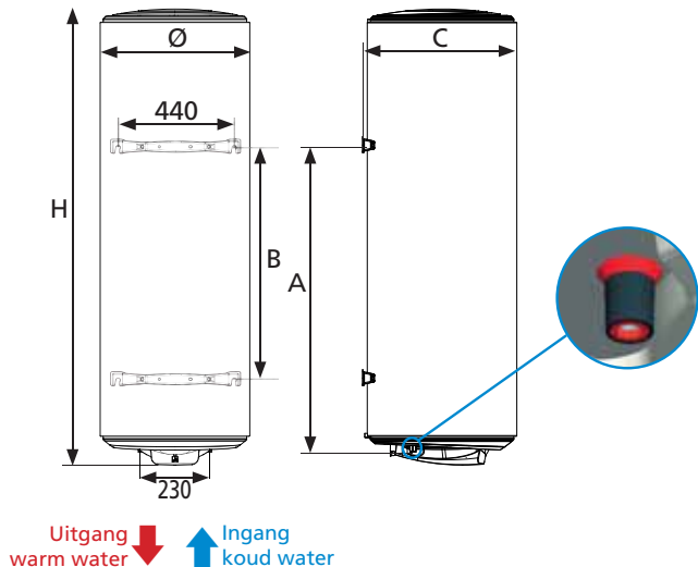
Schematische weergave
